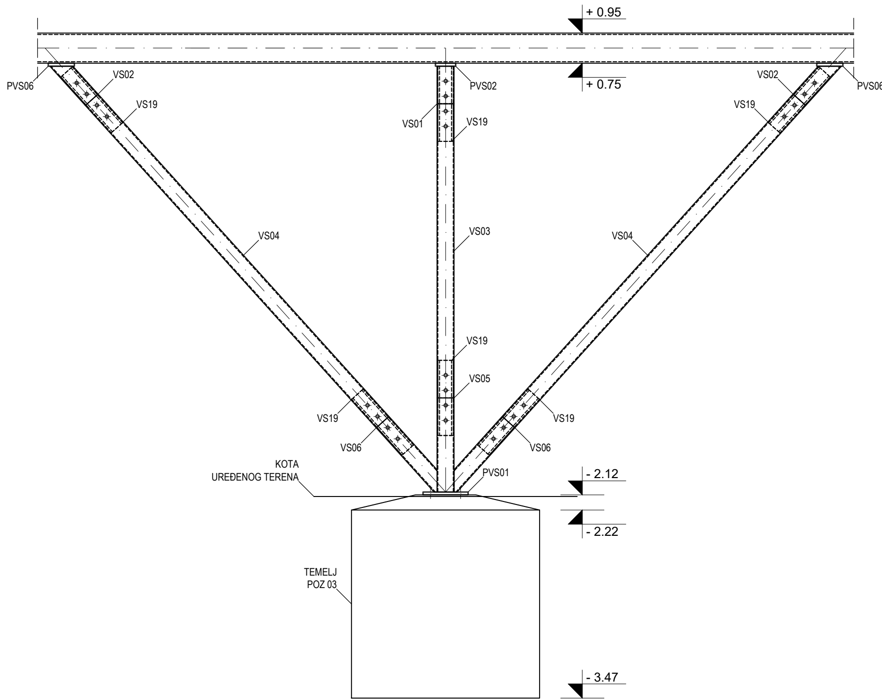
RAZVIJENI PRESJEK 1 - 1
