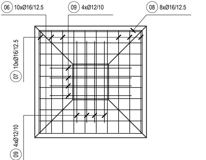
PLAN ARMATURE TEMELJA POZ 03 MJ 1:25
