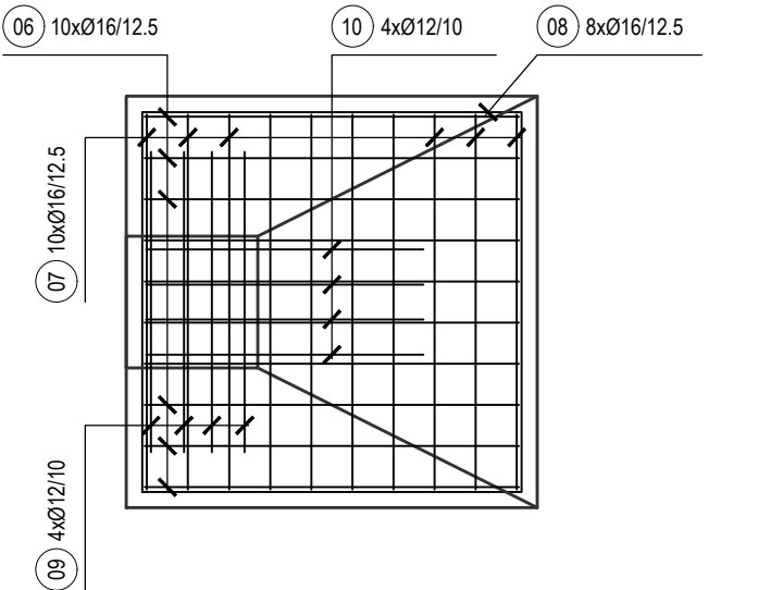
PLAN ARMATURE TEMELJA POZ 02 MJ 1:25
