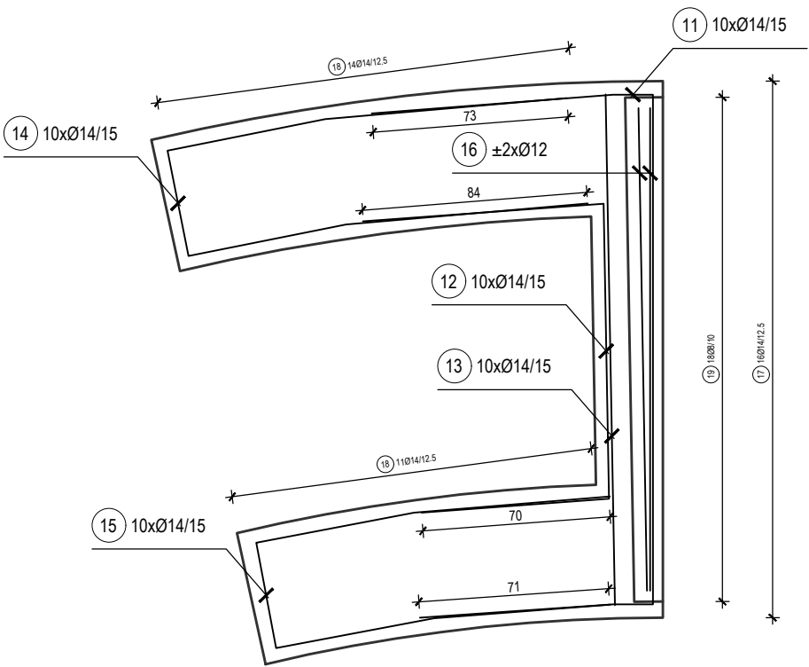
PLAN ARMATURE TEMELJA POZ 04 MJ 1:25
